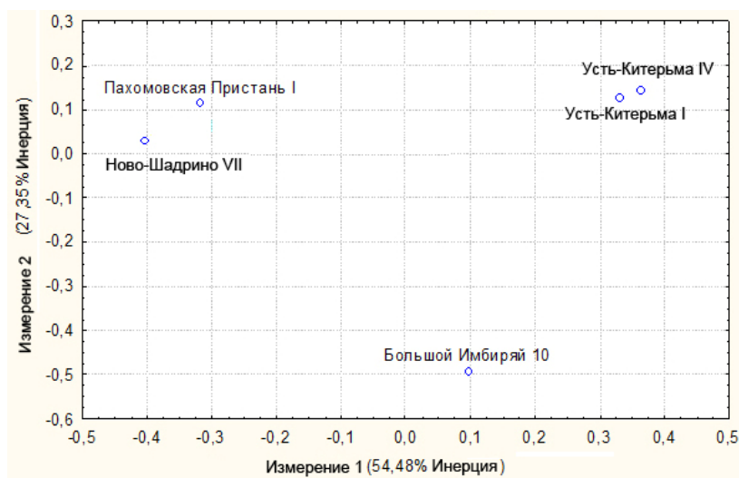
Рис. 2. Двухмерный график анализа соответствий керамики поселений пахомовской культуры
